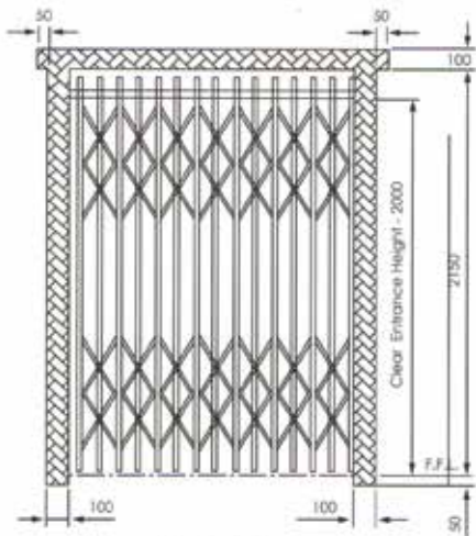
Manual Collapsible Door
